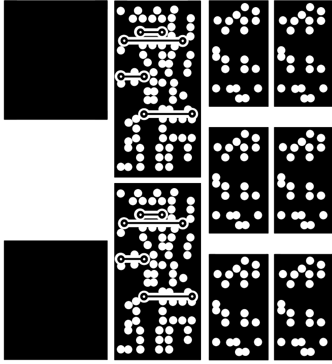
małe płytki - strona masy rysunek lustrzany
