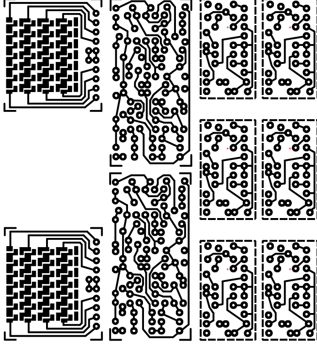
małe płytki - strona elementów rysunek prosty
